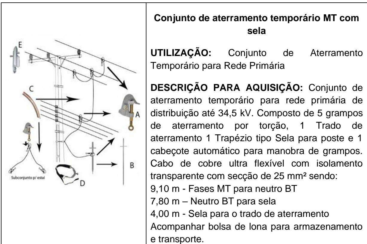
Figura 94 – Conjunto de aterramento temporário MT
