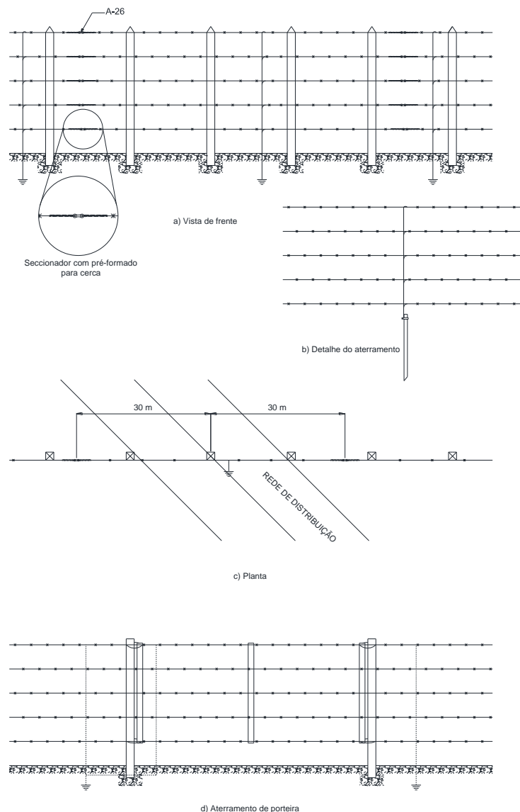
Figura 110 – Seccionamento de cerca – Cerca paralela
