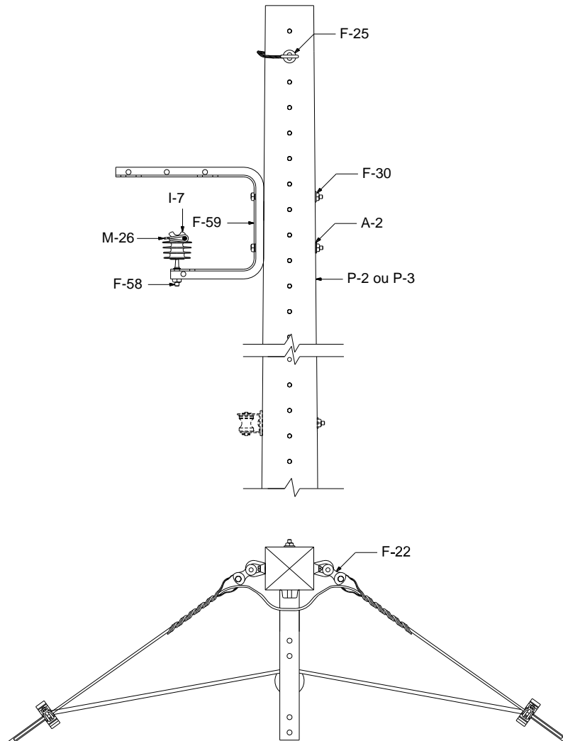
Figura 22 – Estrutura CU2 – Poste de seção DT ou de madeira
