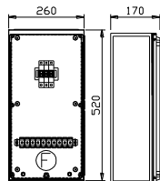
CAIXA PARA BARRA DE EQUIPOTENCIALIZAÇÃO PRINCIPAL (BEP) TIPO (POLIMÉRICO)
