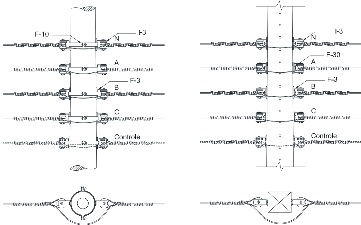
Figura 88 – Estrutura S4
