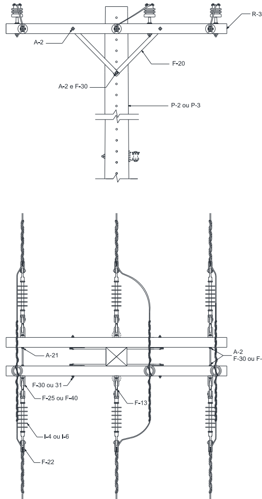
Figura 46 – Estrutura N4 – Poste de seção DT ou de madeira
