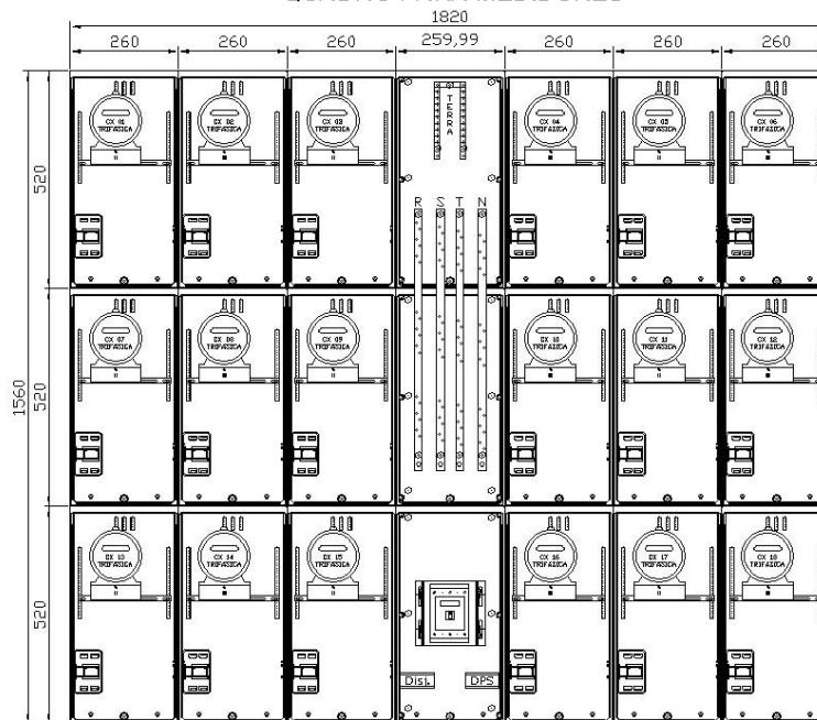
Medição Direta até 175A
