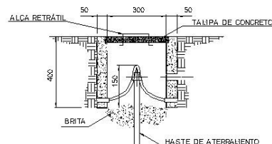
CORTE AA'
