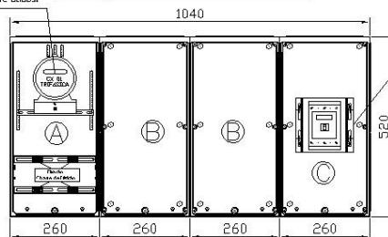
Medição Indireta até 450A
