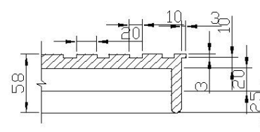
DETALHE — B
